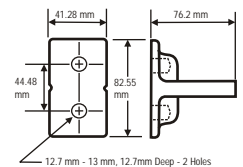
Drwg. A : HCCP - 2120
