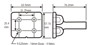
Drwg. C : HCCPL - 4240
