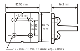
Drwg. B : HCCP - 4120 / HCCP - 4240
